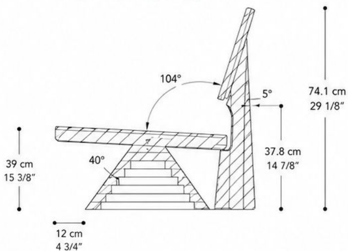
VISTA LATERAL (CORTE)
